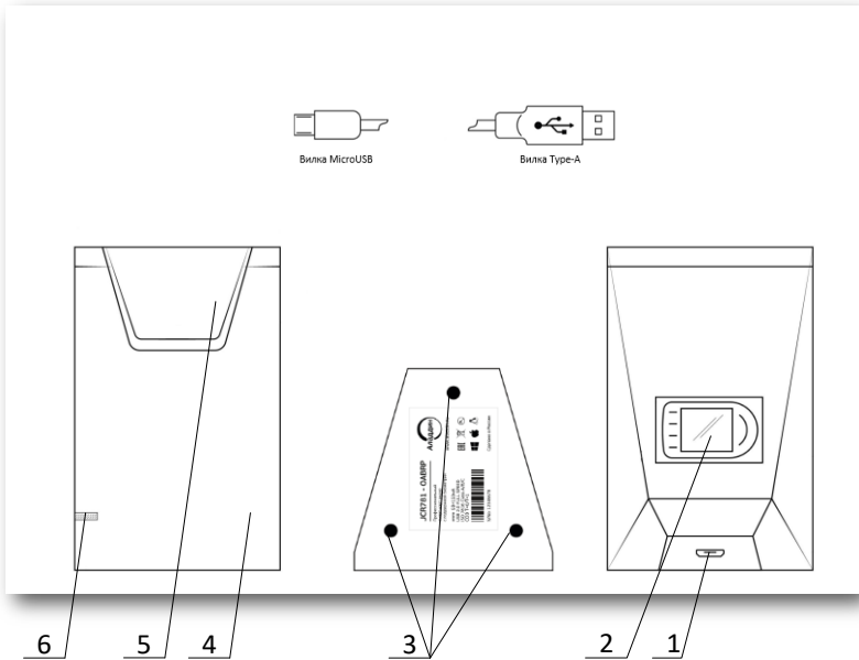
Рисунок 1 – Схема изделия
