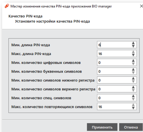
Рисунок 36 — Окно [Мастер изменения качества PIN-кода приложения BIO manager]
