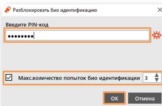
Рисунок 41 — Окно [Разблокировать био идентификацию]
