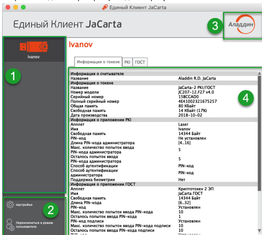
Рисунок 5 – Основное окно Единого Клиента JaCarta в режиме администратора
