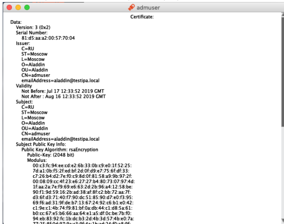
Рисунок 40 – Окно просмотра сертификата
