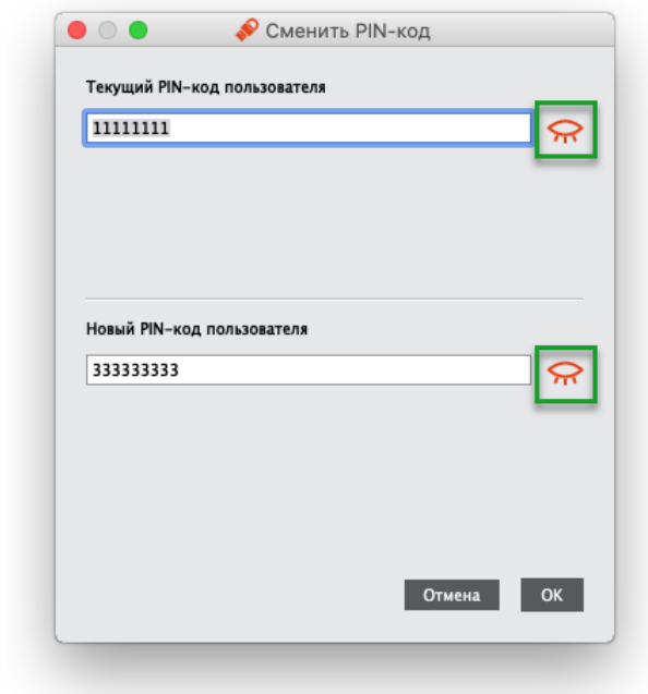
Рисунок 14 – Значения текущего и нового PIN-кода могут быть отображены в явном виде
