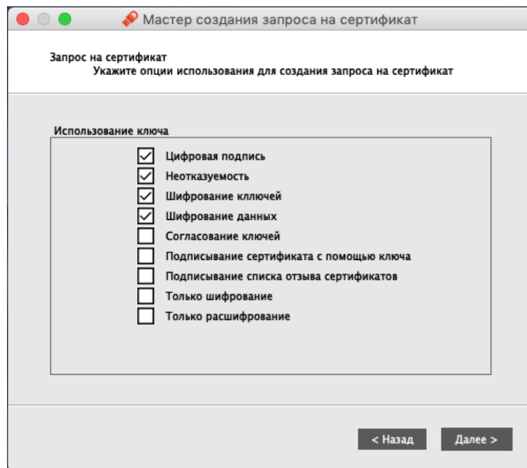
Рисунок 33 - Мастер создания запроса на сертификат. Опции использования ключа
