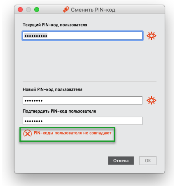
Рисунок 13 – Значения нового PIN-кода не совпадают, поэтому операция не может быть продолжена (кнопка "OK" не активна)
