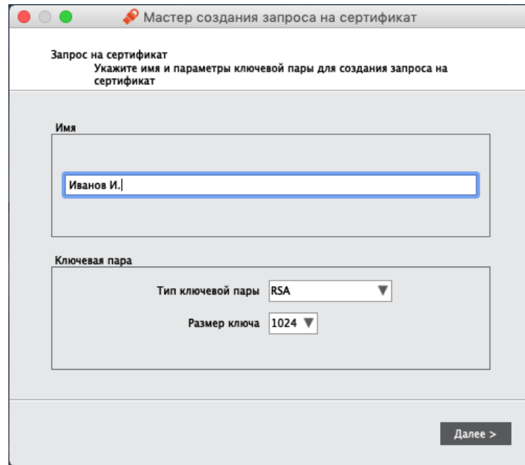
Рисунок 31 - Мастер создания запроса на сертификат. Ввод имени и параметров ключевой пары
