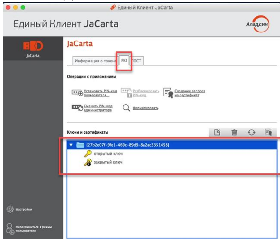
Рисунок 38 - Единый Клиент JaCarta. Полный список объектов в памяти электронного ключа
